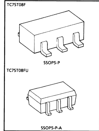
Weight SSOP5-P : 0.016g (Typ.) SSOP5-P-A : 0.006g (Typ.)
